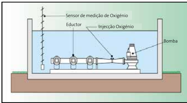
Sistema de Arejamento Halia® de instalação direta
