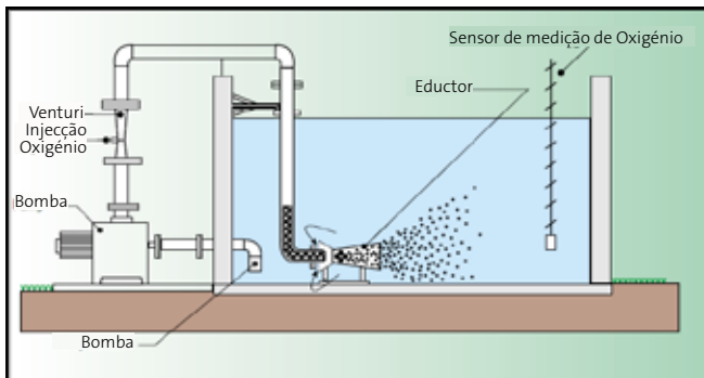
Sistema de Arejamento Halia® de instalação fixa
